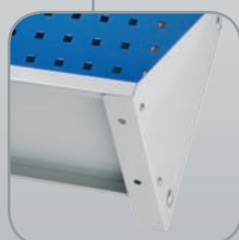
*RasterPlan Stellwände sind generell mit verdeckten Anschraublöchern zur Bodenverankerung vorbereitet.
