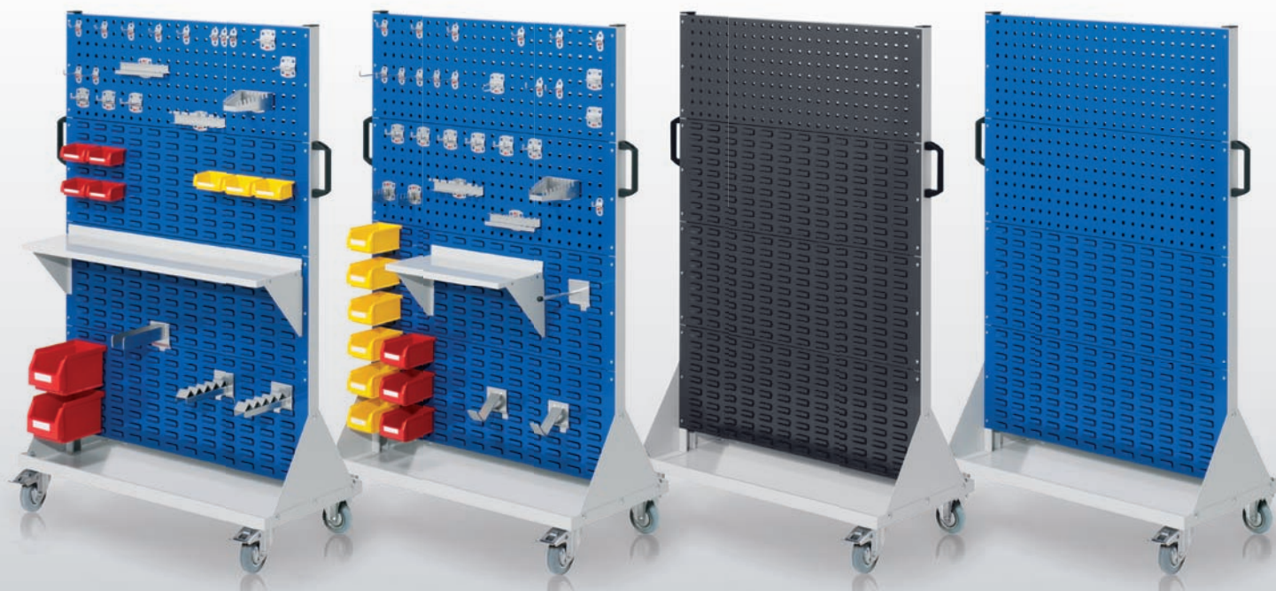
RasterMobil® Größe 4 - H 1580 x B 1000 x T 500 mm
