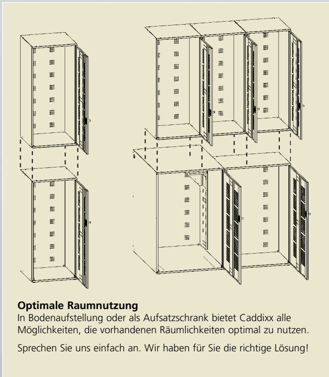
Einzel-Caddieschrank Zur Unterbringung eines Ziehcaddies. Für Bodenaufstellung oder als Aufsatzschrank. Mit rechts oder links angeschlagenen Türen je nach Aufstellung.
