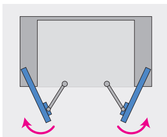
Funktionsprinzip Einschwenktüren.
