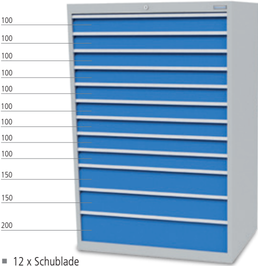
■ 12 x Schublade
