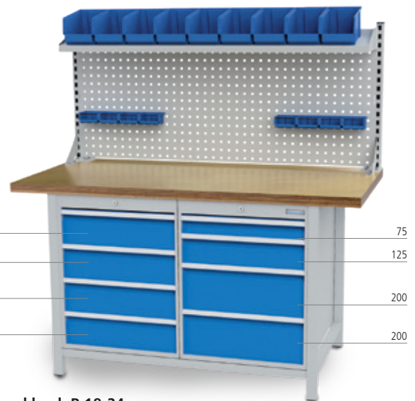
Kastenwerkbank R 18-24
