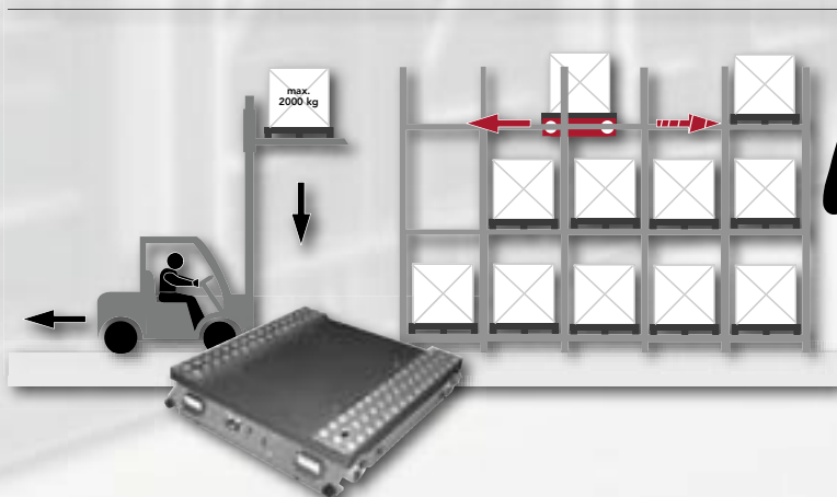
Autosat – automatischer Satelliten-Förderer zur Palettenverschiebung; First-in-First-out oder First-in-Last-out, je nach Logistikkonzept
