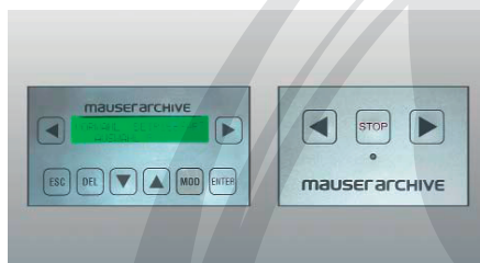
links Programmierbares Bedienfeld; Steuereinheit mit Display rechts Bedienfeld «Regalachse» Links-/Rechts- und Stopptaste
