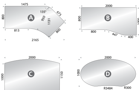
Maßskizzen mit BAP rechts
