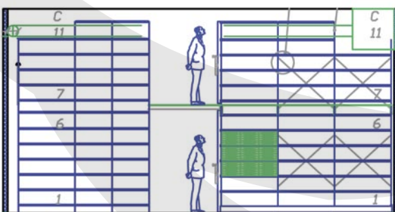
Ansicht: Planung Erdgeschoss
