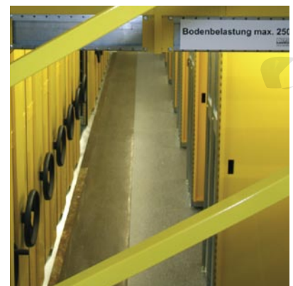
Ansicht Erdgeschoss: Duplex-Rollregalanlage, Fachbodenregale mit Schiebetüren.
